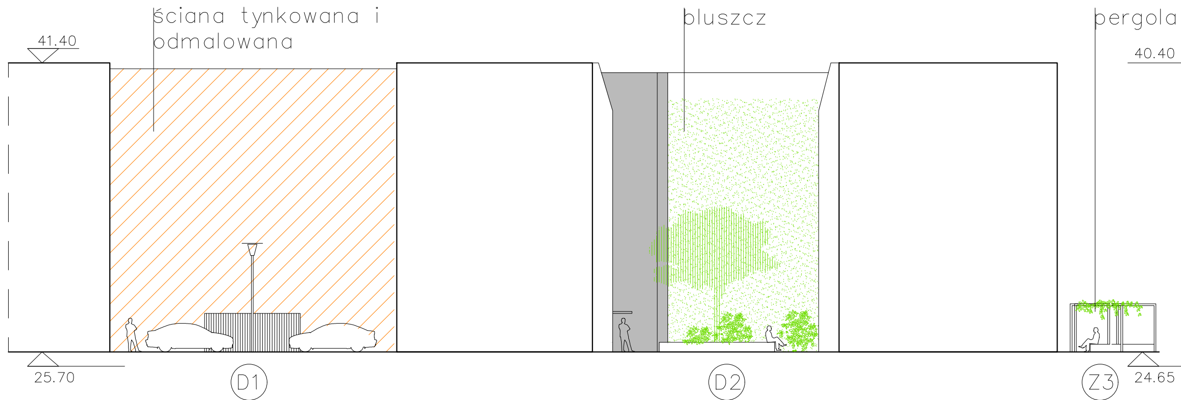
PRZEKROJÓJ BB
